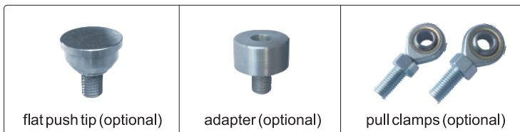
DF2K
